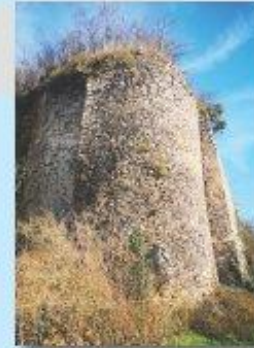
Four à chaux bâti sur un plan de J.-É. Renou à Chaudfontaine-sur-Layon.
